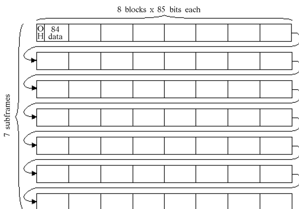
Fig. 18-7. DS-3 / T-3 Multiframe format
