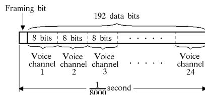
Fig. 18-1. One DS-1 Frame = 193 bits
